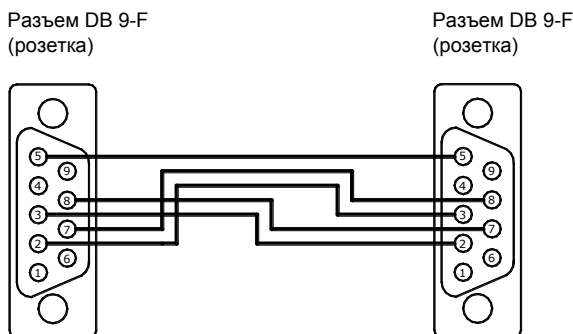
Рис. 9.6 Нуль - модемный кабель RS-232C
