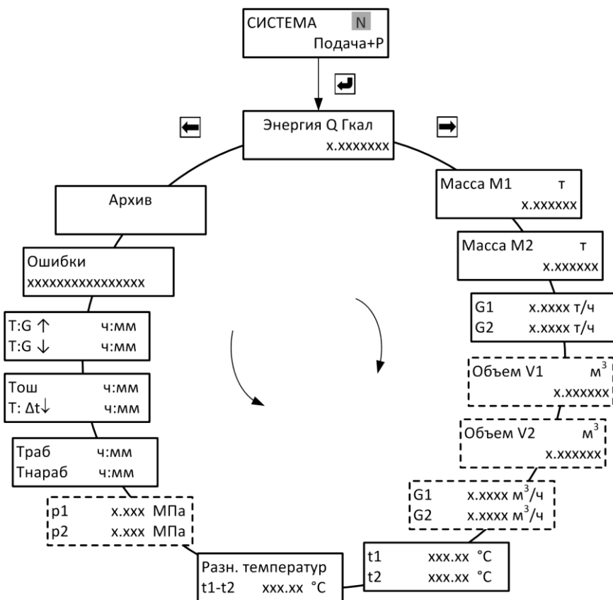
Рис. Г.7 Схема меню режима «Рабочий» для схемы учета «ПОДА-ЧА+P»
