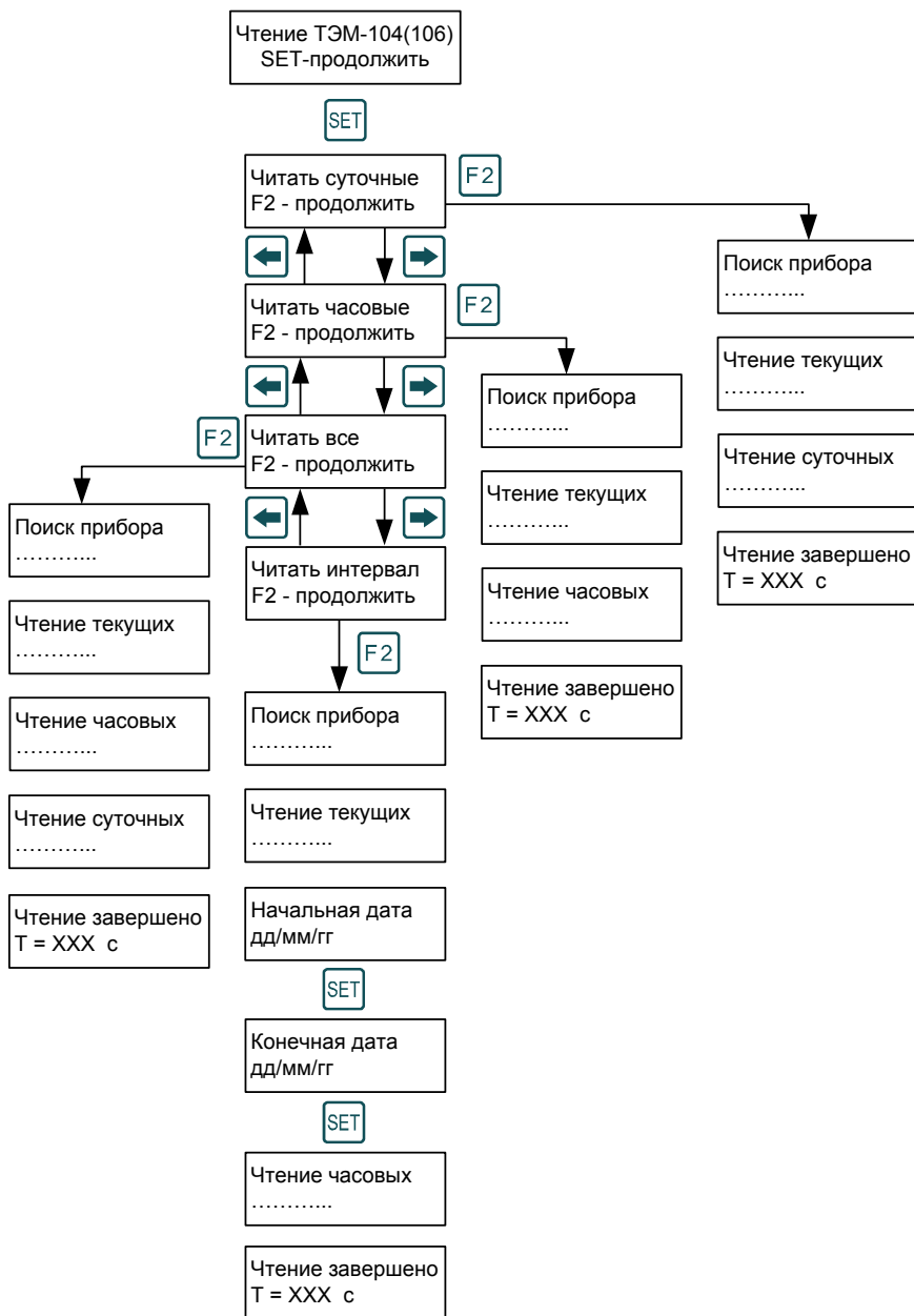
Рис. В.2 Режим чтения данных из теплосчетчиков ТЭМ-106, ТЭСМА-106 и ТЭМ-104
